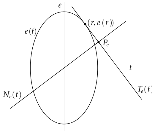
Fig. 2 The ellipse
