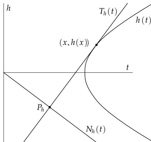
Fig. 1 The hyperbola
